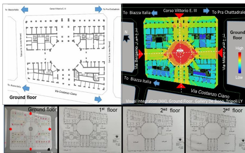
الشكل رقم (8): اعلي يسار: المسقط الأفقي للطابق الأرضي (المصدر: إعادة رسم من طرف المؤلف بناء على صورة للمسقط 2026)، ويمينه التكامل البصري النحوي المكانى Visual Integration [HH] (المصدر: المؤلف) وفي الأسفل المساقط الأفقية الأربعة لطوابق مبني رواق الكرامة (De Bono)، (المصدر: صور للمساقط الأفقية بالمبنى خلال الصيانة، يوليو 2026). ملاحظة: ان تسميات الشوارع بهذه الخرائط هي "September street" و "Imhmmid al Mmqaryif street" وعنوان الخرائط "غاليريا دي بونو" — رواق الكرامة، مجموعة اليقين القابضة Al Yaqeen Holding Group.
